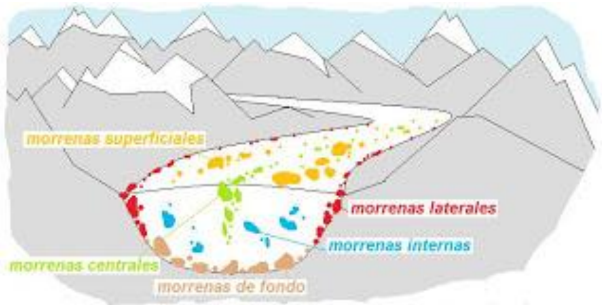
corte transversal de una lengua de glaciar
