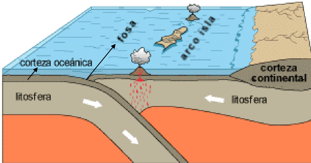
Convergencia corteza oceánica - corteza oceánica
