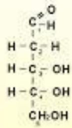
D - Desoxirribosa
