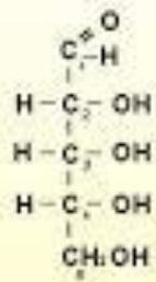
D - Ribosa
